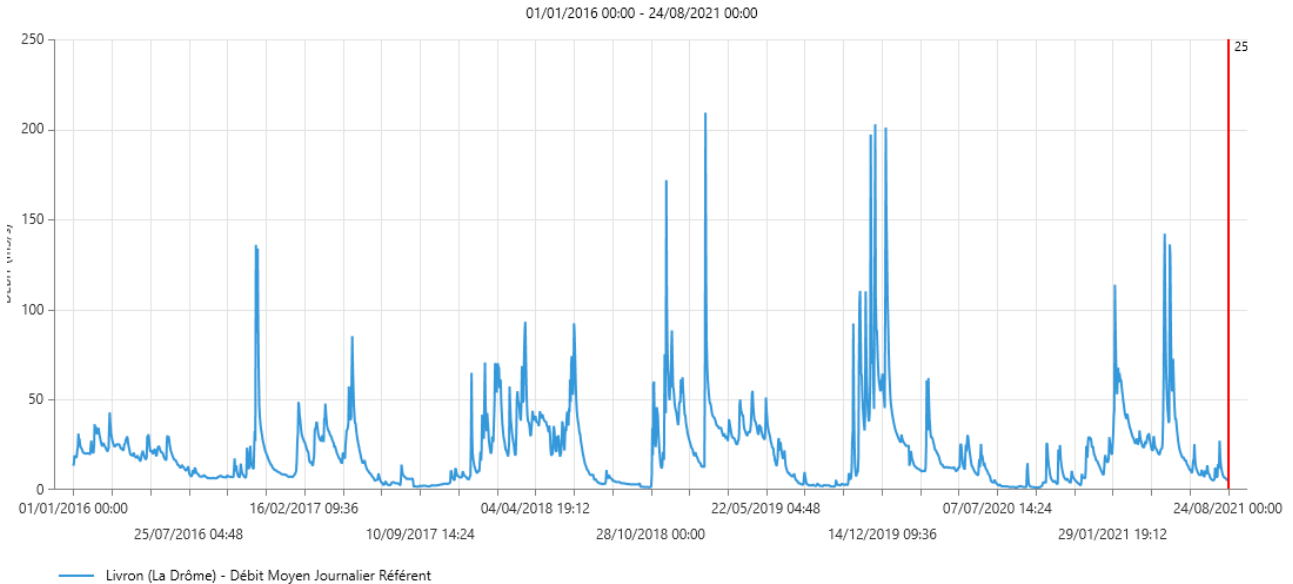
Figure 7 : Débit moyen journalier de la Drôme à Livron entre 2016 et 2021 (pour mémoire les débits caractéristiques sont les suivants : Module = 17 m 3 /s, Q2 = 190 m 3 /s, Q5 = 290 m 3 /s).
