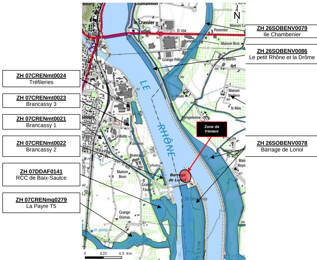
Figure 10. Localisation des zones humides d'après IGN25. © DatARA 2018
