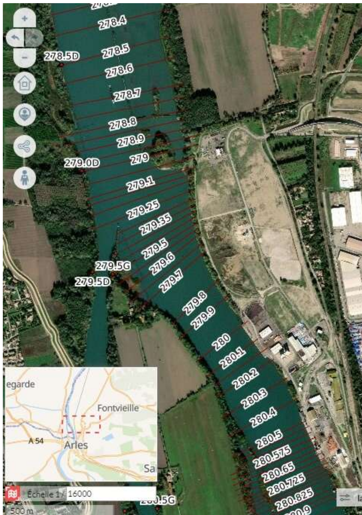
Figure 30. Vue en plan globale du site – Identification des principaux profils entre 278.300 et 280.900 (CNR 2020)
