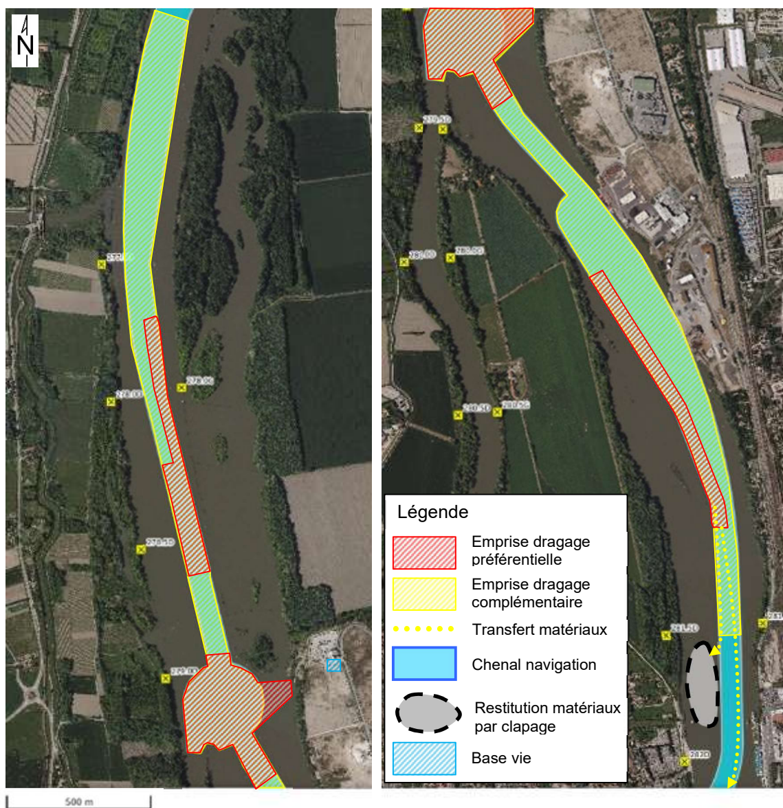
Figure 2. Localisation des travaux (© IGN - CNR 2026)
