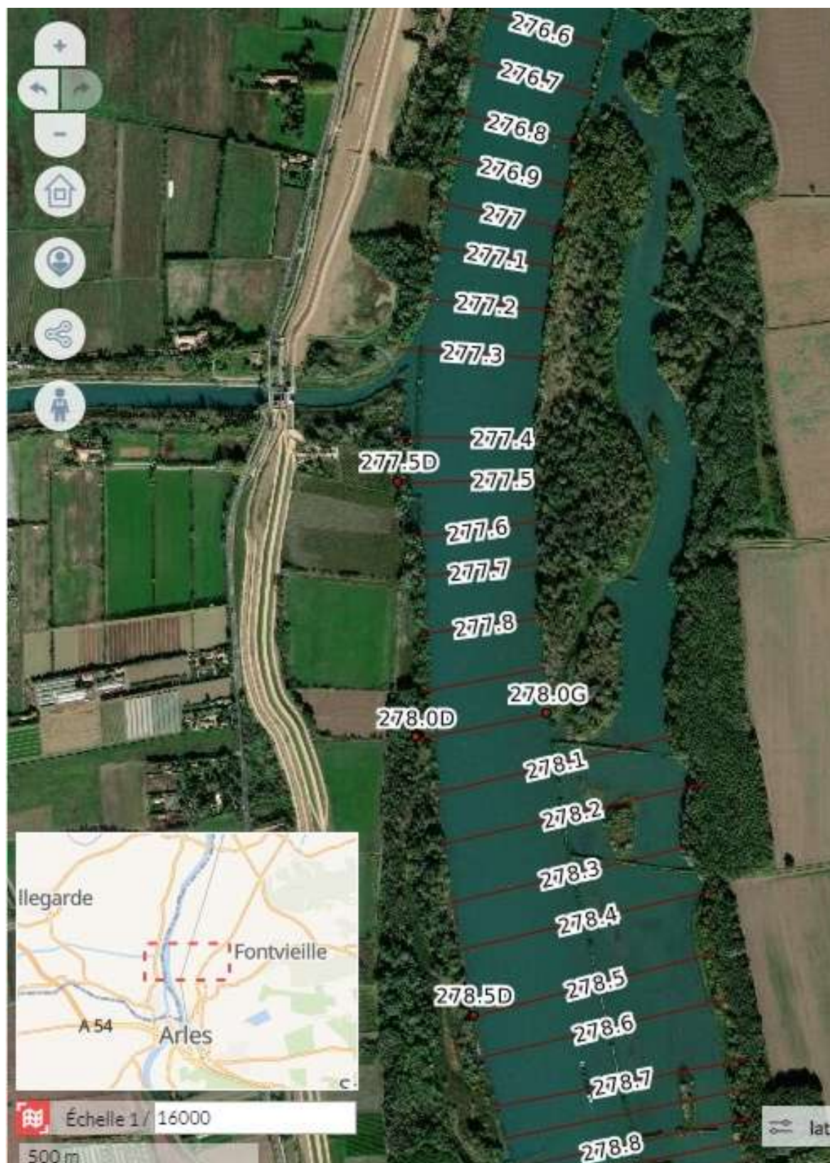
Figure 29. Vue en plan globale du site – Identification des principaux profils entre 276.600 et 278.800 (CNR 2020)
