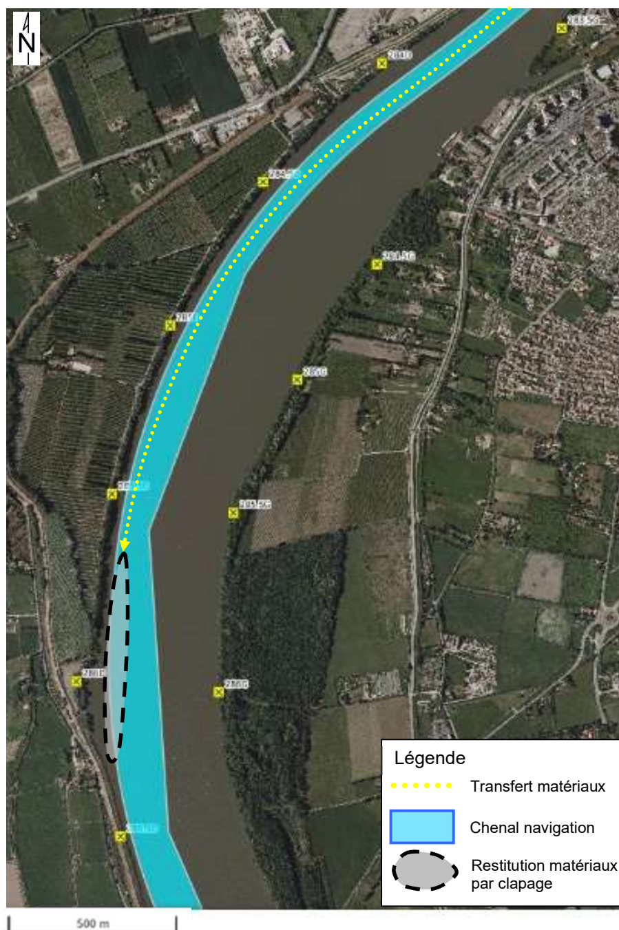
Figure 2 bis. Localisation des travaux (© IGN - CNR 2023)
