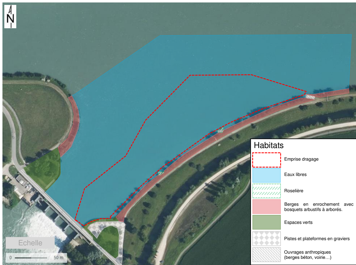
Figure 7. Localisation des habitats dans l'emprise de dragage en amont du barrage de Champagneux (Géoportail 2023).
