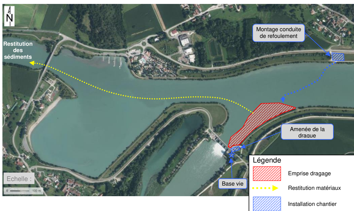
Figure 2. Localisation des travaux (© Géoportail 2022)
