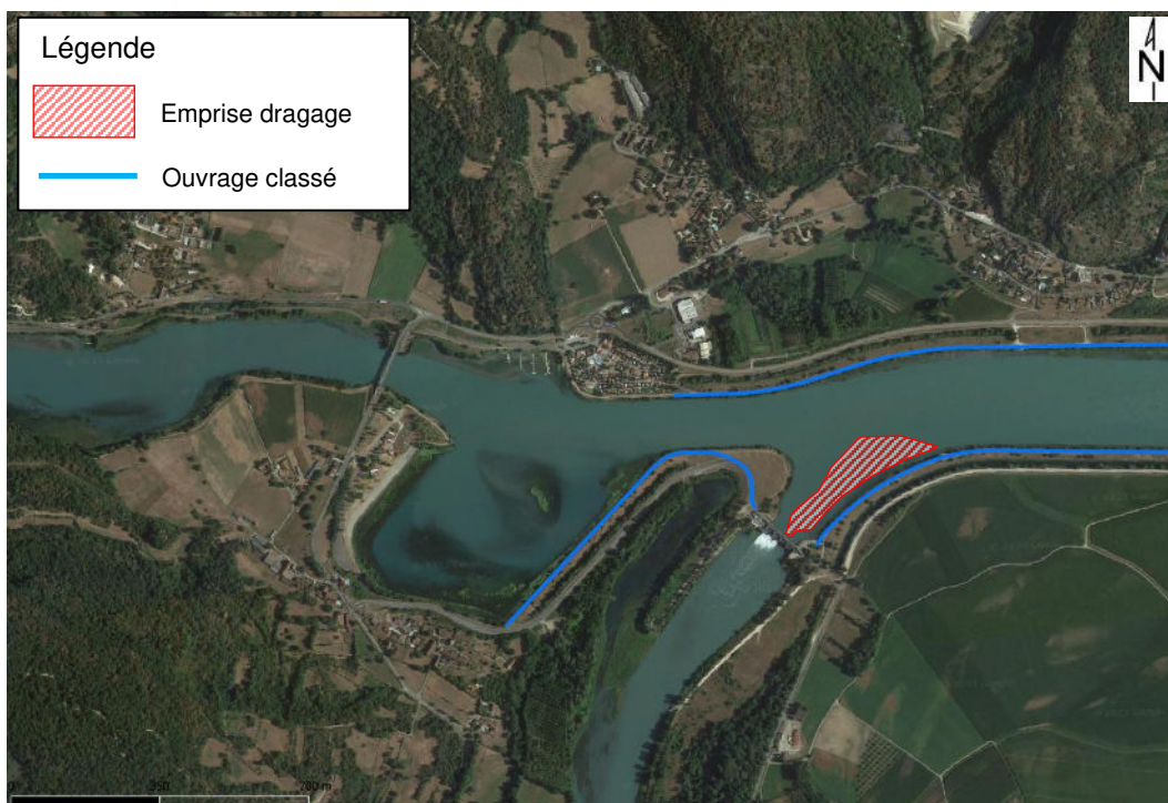
Figure 20. Ouvrages classés à proximité des travaux (CNR 2023)
