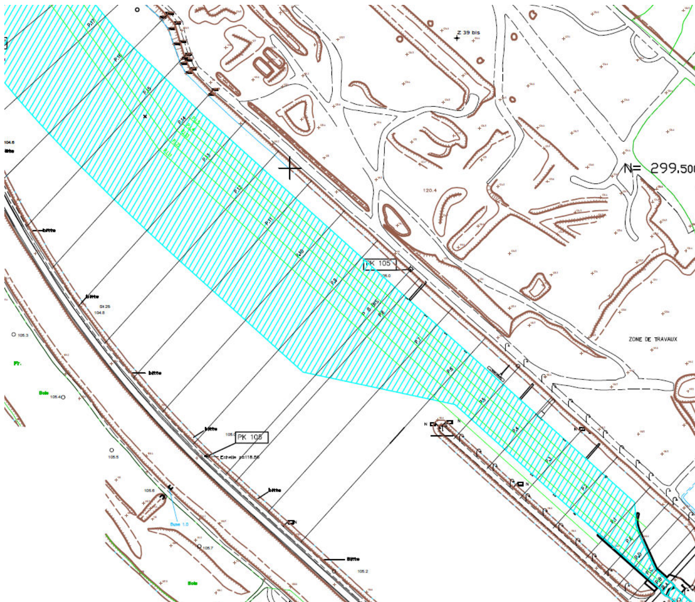
Figure 14. Vue en plan globale du garage amont de Bourg-lès-Valence– Identification des principaux profils entre PA et P16 (CNR 2021)
