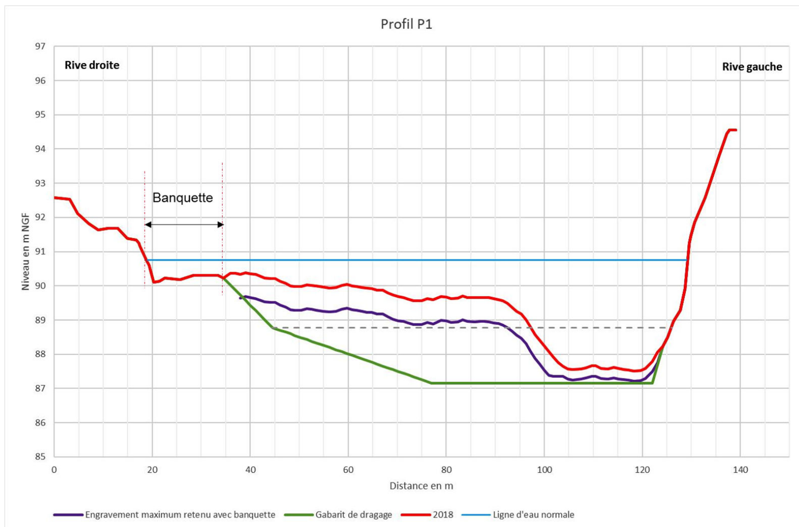
Figure 21. Profil en travers P1 avec gabarit de dragage réduit pour conservation d'une banquette en rive droite
