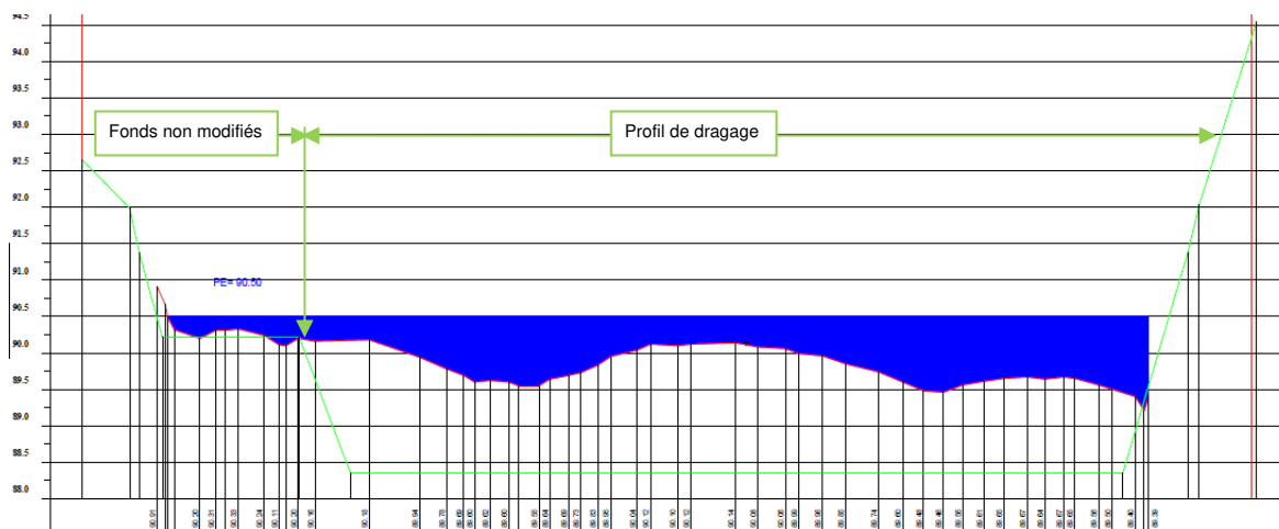
Figure 3. Profil de dragage au profil 9 avec préservation d'une banquette de 15 m vue vers l'amont (CNR 2017)
