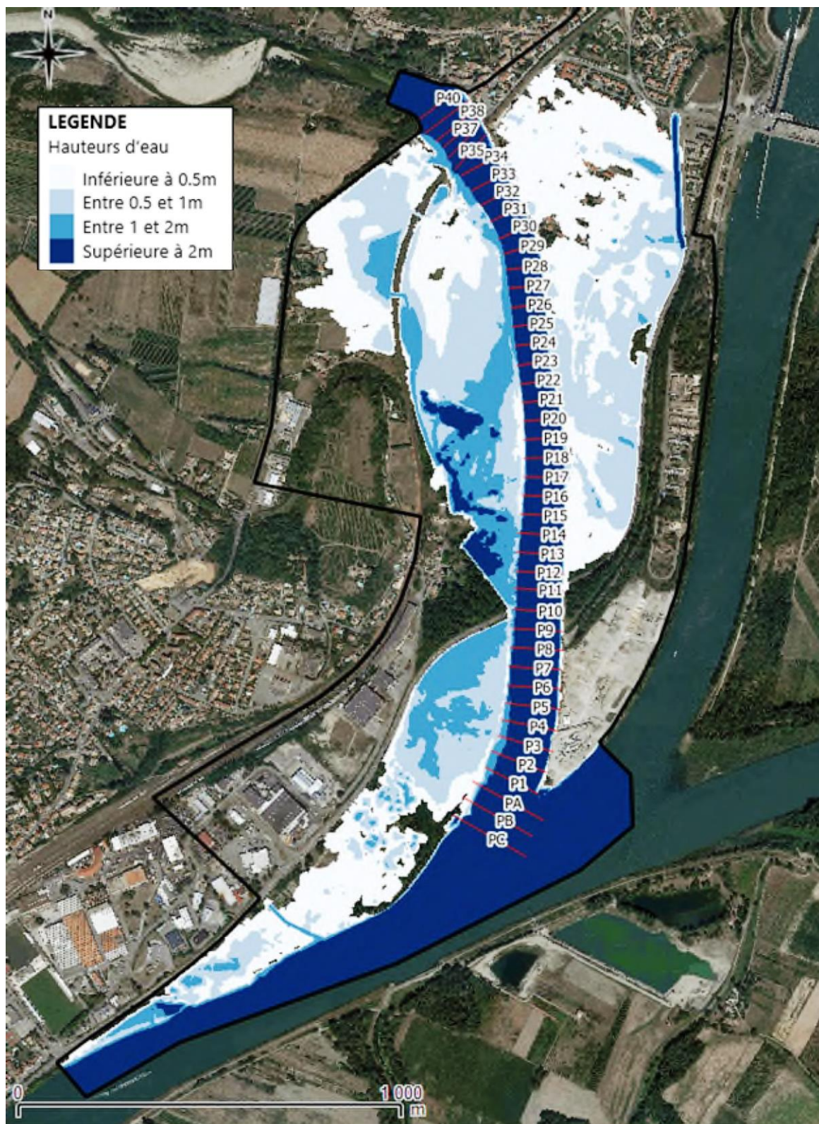
Figure 20. Champ d'inondation de l'Eyrieux pour une crue de 1 500 m³/s.
