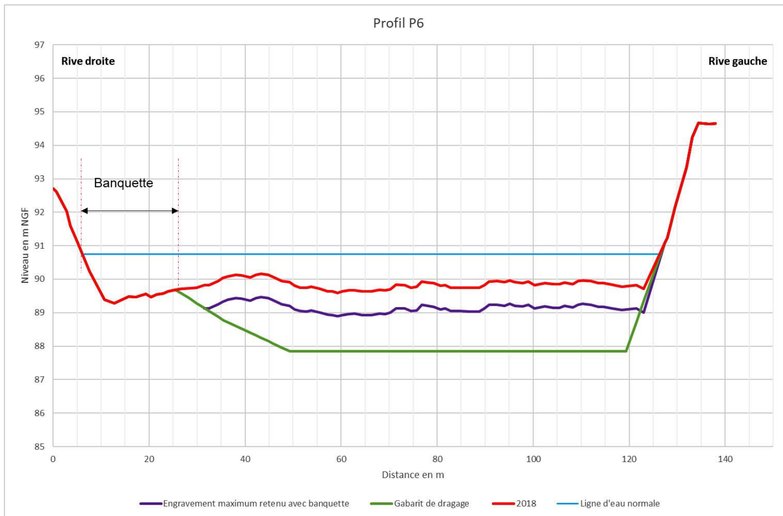
Figure 22. Profil en travers P6 avec gabarit de dragage réduit pour conservation d'une banquette en rive droite
