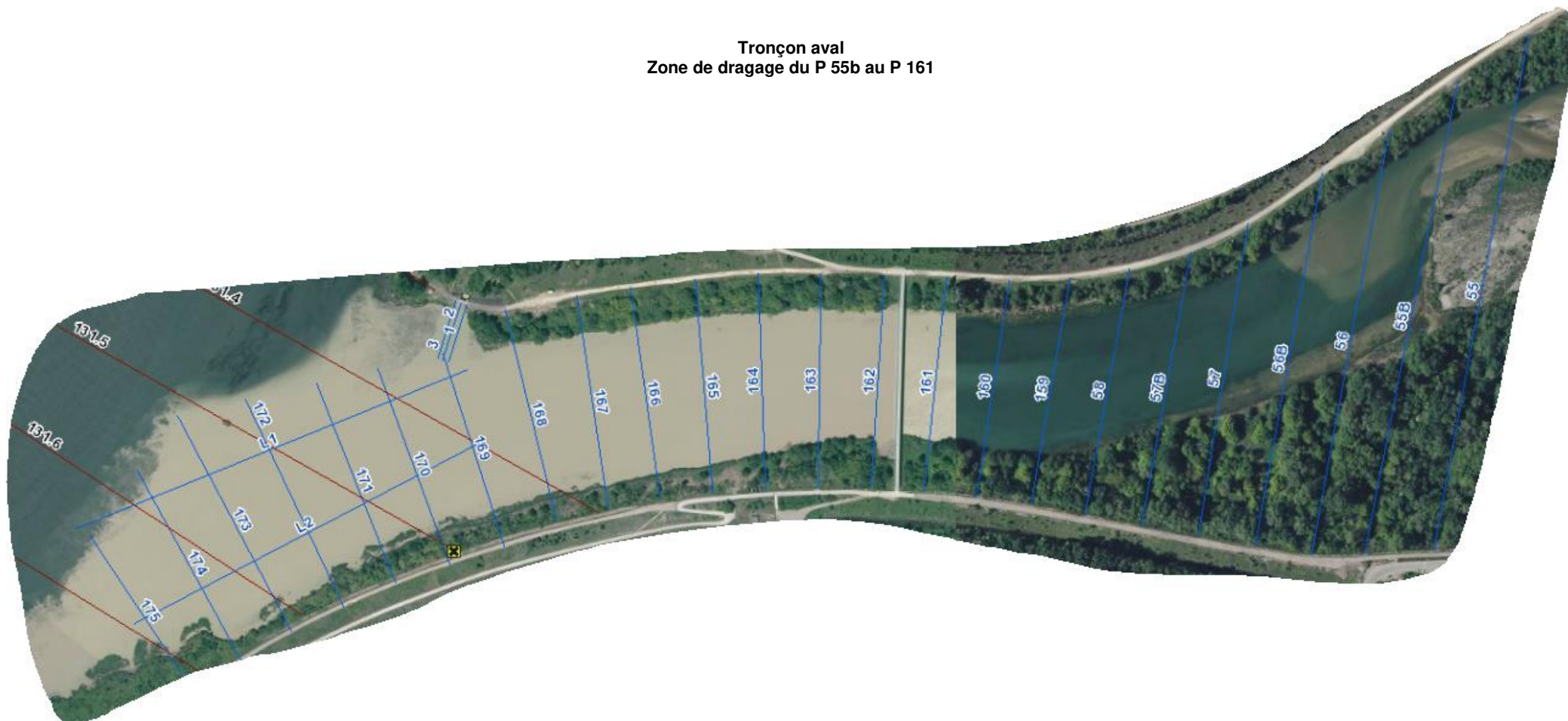
Figure 23. Tronçon aval de la confluence de la Drôme – Localisation des profils (CNR 2019)
